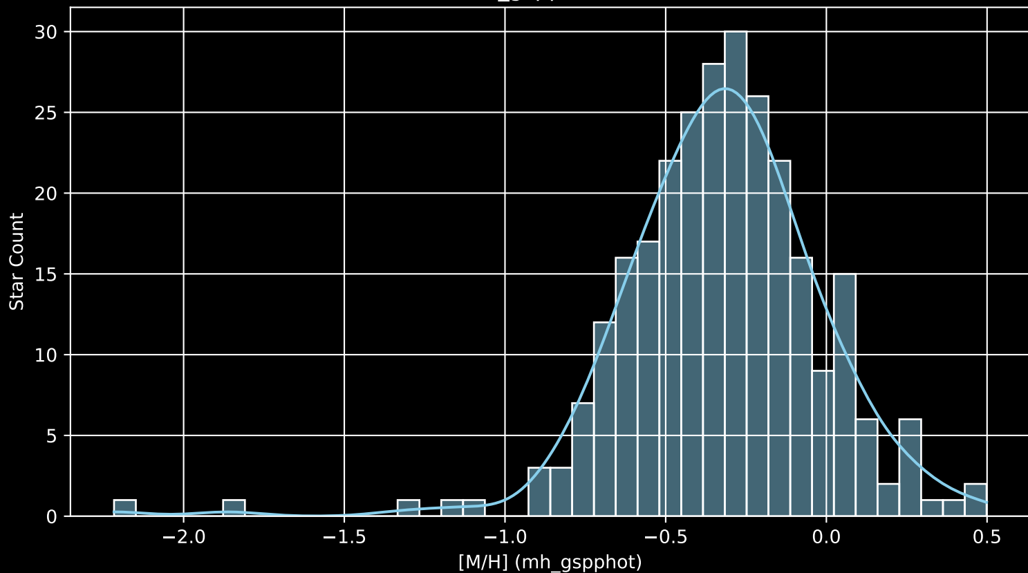
GALAH DR4 Field: [1326] [M/H] (mh_gspphot) (n= 274)
