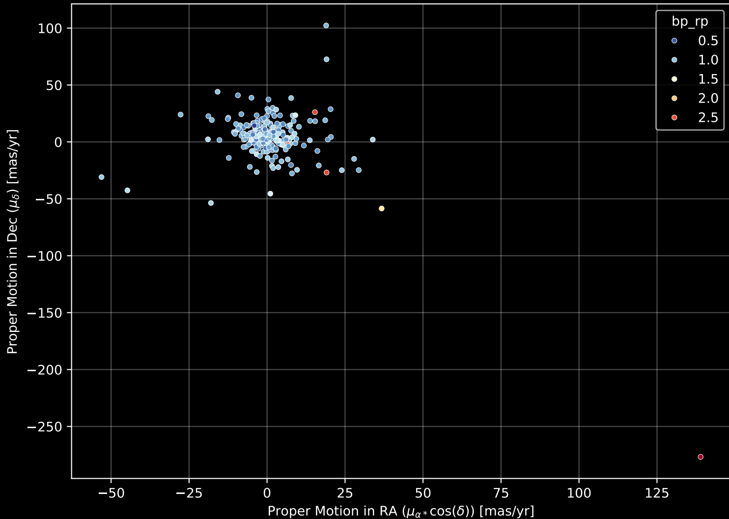
GALAH DR4 Field: [1326] Proper Motion Diagram (n= 274)
