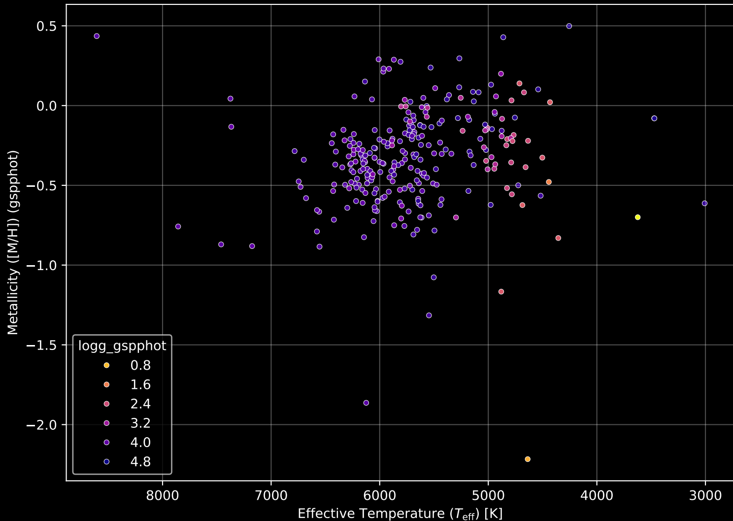
GALAH DR4 Field: [1326] Stellar Population Parameters (n= 274)
