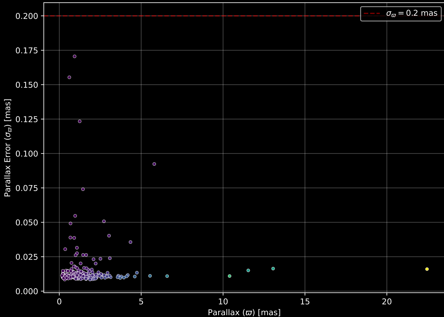
GALAH DR4 Field: [1326] Parallax Quality (n= 274)
